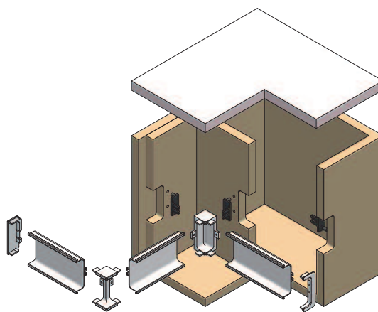
horizontální zásuvkový "C" profil
