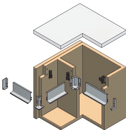
horizontální dvířkový "J" profil
